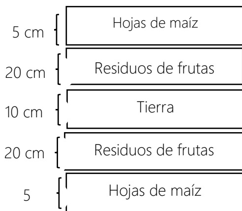
Figura 2. Conformación de la pila
