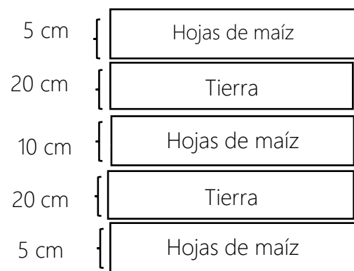
Figura 4. Conformación de la pila de compost.
