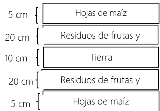
Figura 3. Conformación de la pila de compost
